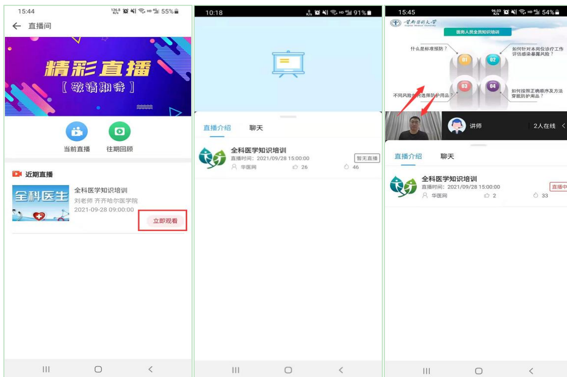
直播列表
